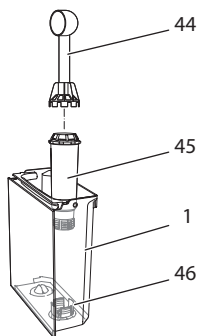
Fig. 24: Vissage/dévisage du filtre à eau
