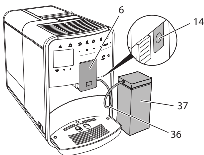
Fig. 12: Collegamento del serbatoio del latte alla macchina da caffè
