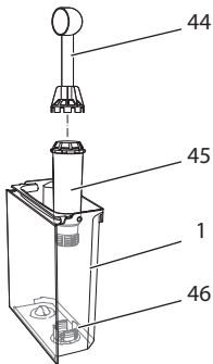
Abb. 24: Wasserfilter ein-/ ausschrauben
