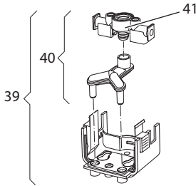
Abb. 23: Milcheinheit ausbauen
