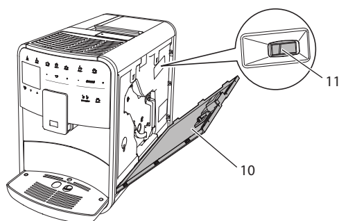
Fig. 20: Regolazione del grado di macinazione
