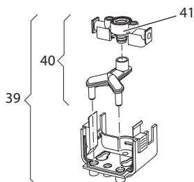
Afb. 23: Melkeenheid demonteren
