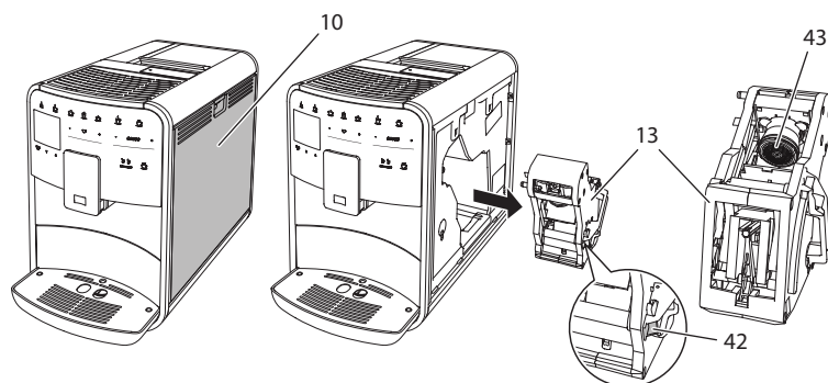
Abb. 22: Brühgruppe ausbauen
