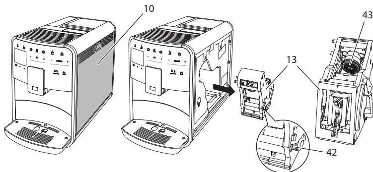
Fig. 22: Smontaggio dell'unità bollitore
