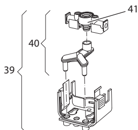
Fig. 23: Smontaggio del gruppo latte
