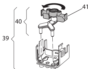
Afb. 21: Toevoer draaien
