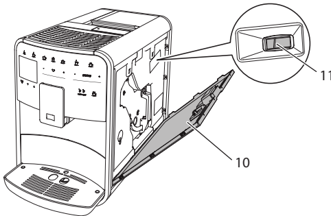
Abb. 20: Mahlgrad einstellen
