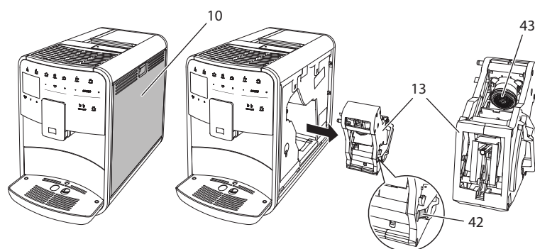
Afb. 22: Zetgroep demonteren
