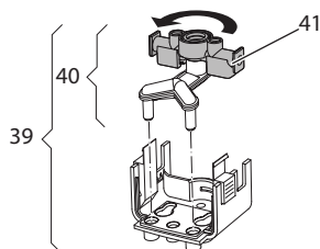
Fig. 21: Rotazione del tubo di mandata latte
