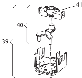
Fig. 23: Démontage du groupe lait
